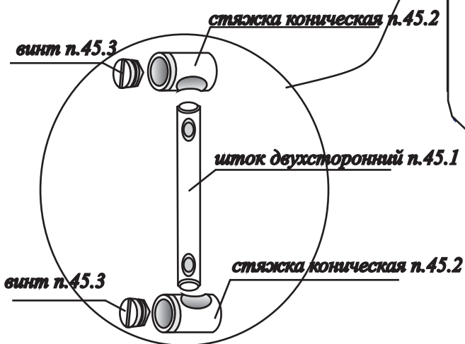
Рис.24 (Поз.№ 45 стяжка коническая двухсторонняя в сборе)
